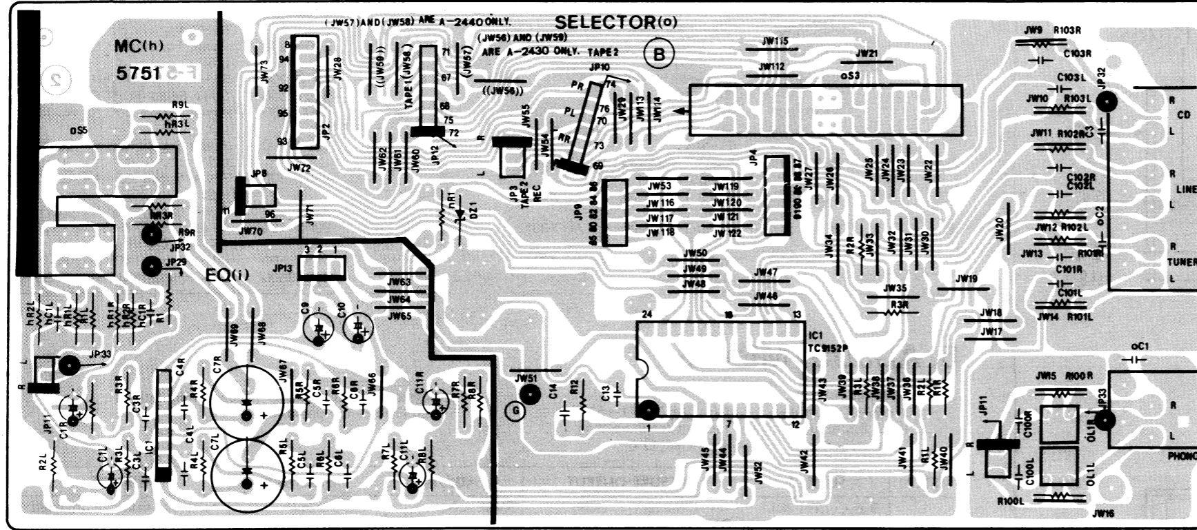
3-6. F-5751 EQ Amp. & INPUT Terminal Board
