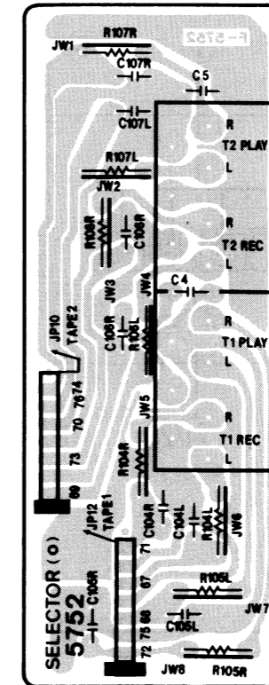
3-8. F-5752 TAPE/DAT
